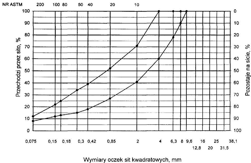
Rys. 3. Krzywe graniczne uziarnienia mieszanki mineralnej BA od 0 do 6,3 mm, od 0 do 6,3 mm do warstwy ścieralnej nawierzchni drogi o obciążeniu ruchem nawierzchni drogi o obciążeniu ruchem KR1 lub KR2
